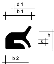
Form C / LKDC - Deckel / cover druckloser Behälter / pressless tank
