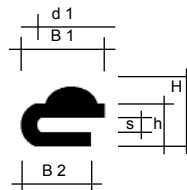
Form A / LKD druckbelasteter Behälter pressurised tank
