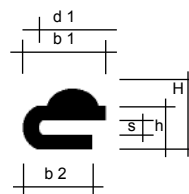
Form A LKD - Deckel / cover druckbelastete Behälter / pressurised tanks
