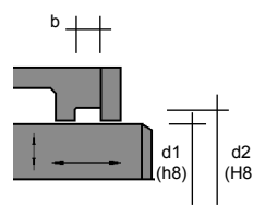
Stangendichtung / rod seal
