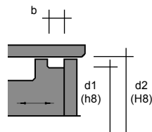
Kolbendichtung / piston seal
