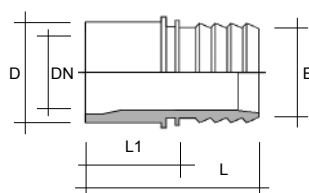
Schlauchstutzen mit Anschweißende / hose shank with butt weld
