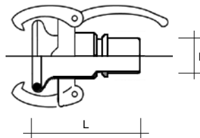
Kupplungen mit Bundstutzen couplings with hose shanks and collar
